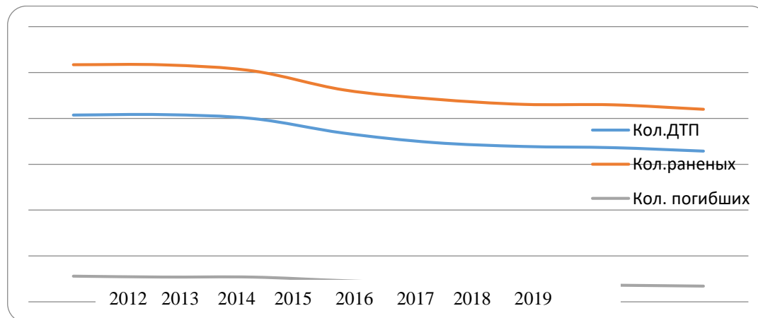
Рисунок 1. Основные показатели аварийности за 2012-2019гг.
