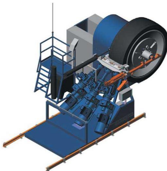
Рис. 4. Опытный образец сборочного станка «Base Constructor для обрезинивания каркасов КГШ и СКГШ» фирмы VMI Group (Голландия).
