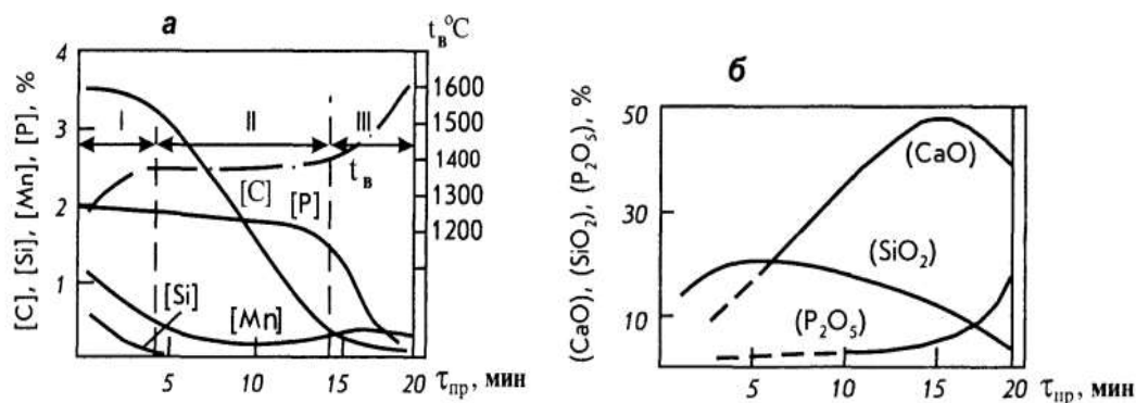
Рисунок 1 – Изменение состава и температуры ванны t (а), состава шлака (б)
